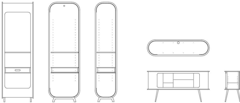
Innenausbau: Tablare verstellbar Auszugskorb verstellbar Innenhöhe: 8 - 13 - 18 cm
